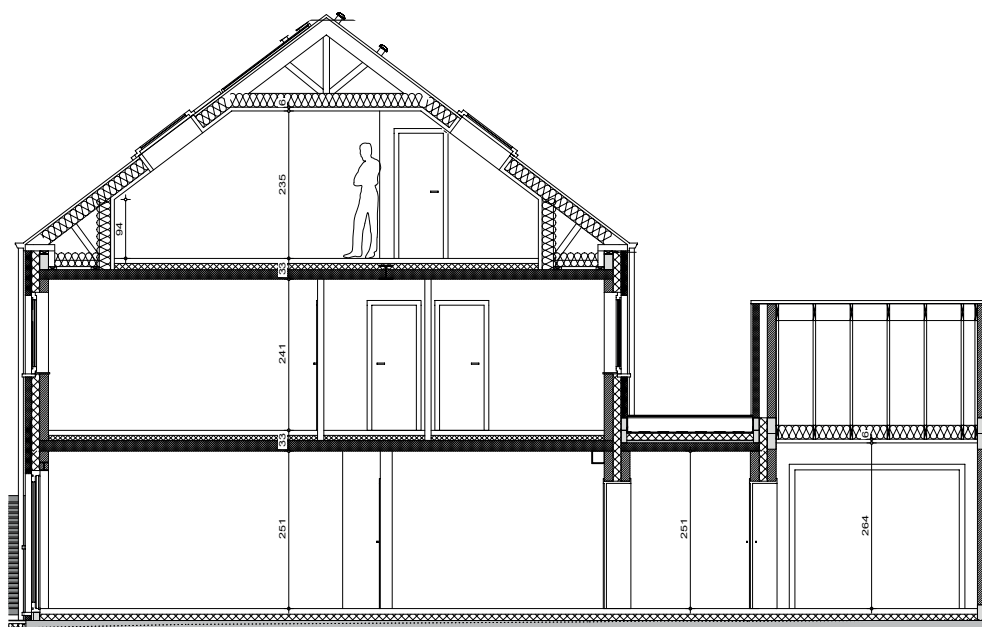
Coupe
